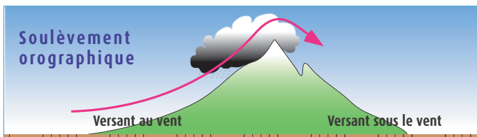
Soulèvement orographique
