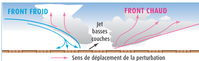
Soulèvement frontal
